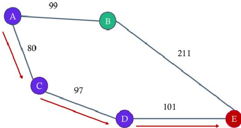
Grafo de Estados y Cola de Prioridad
